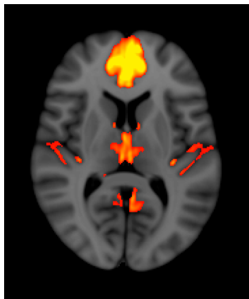
node 14 -0.89
