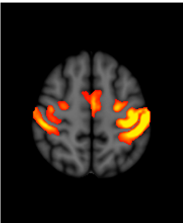
node 11 -1.21
