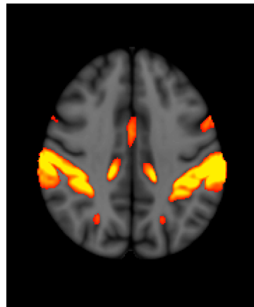
node 7 0.78
