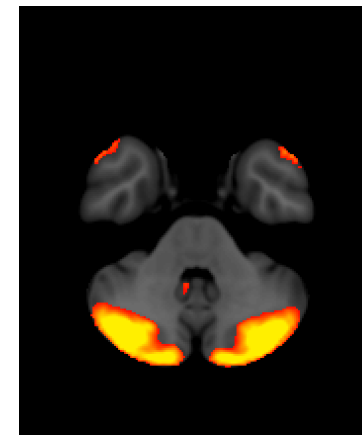
node 1 0.60
