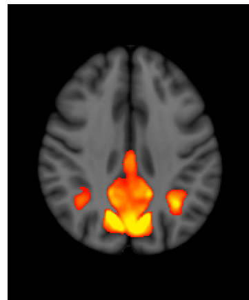
node 20 0.66
