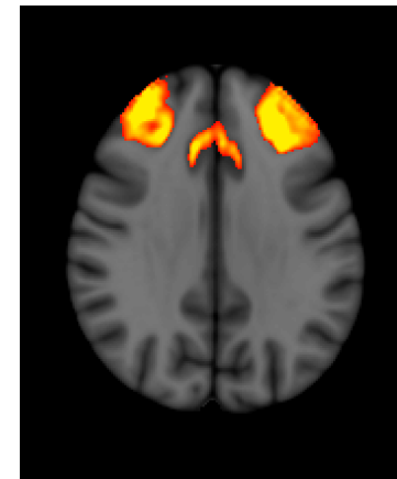
node 5 0.64
